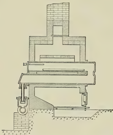
FIG. 102.—Pintsch Gas Retort.
